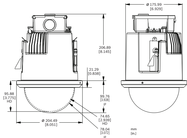
Dimensioni AUTODOME 7000: montaggio a soffitto
